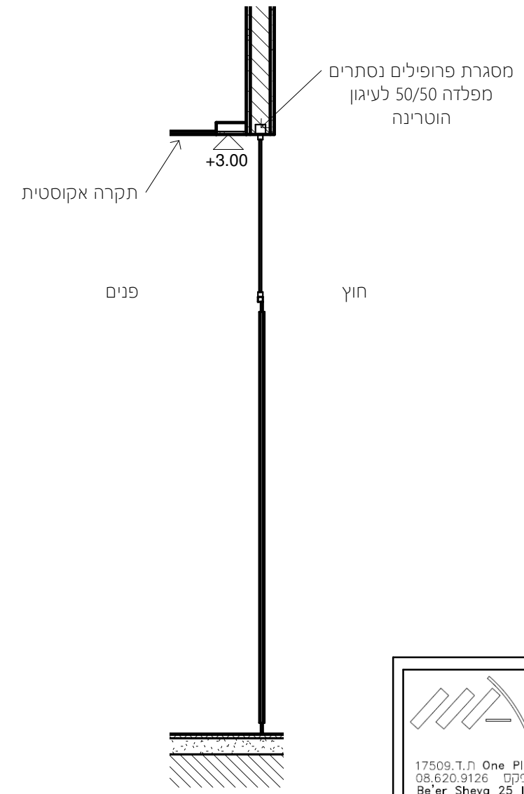
חתך
