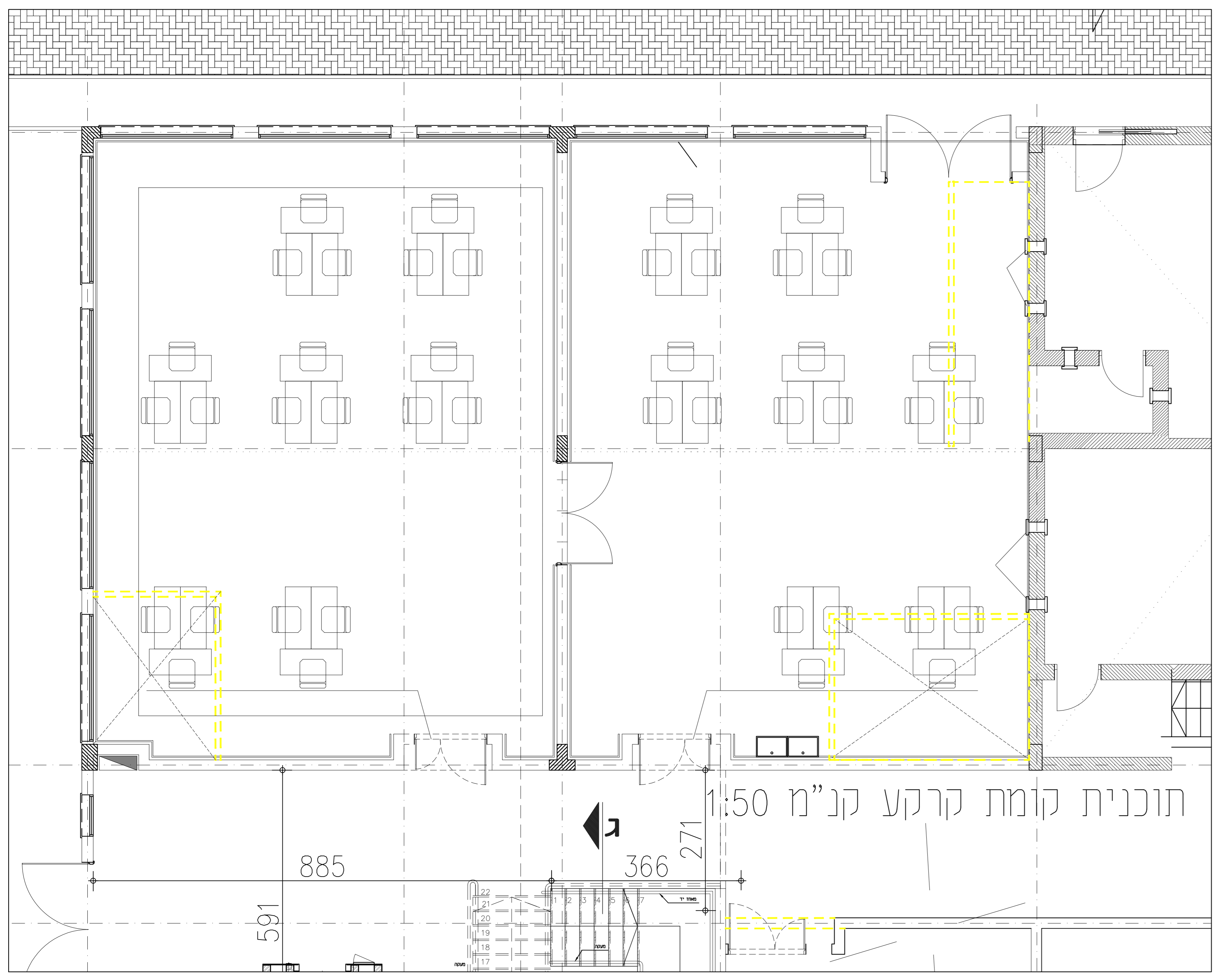
קומה קרקע - העמדת ריהוט
